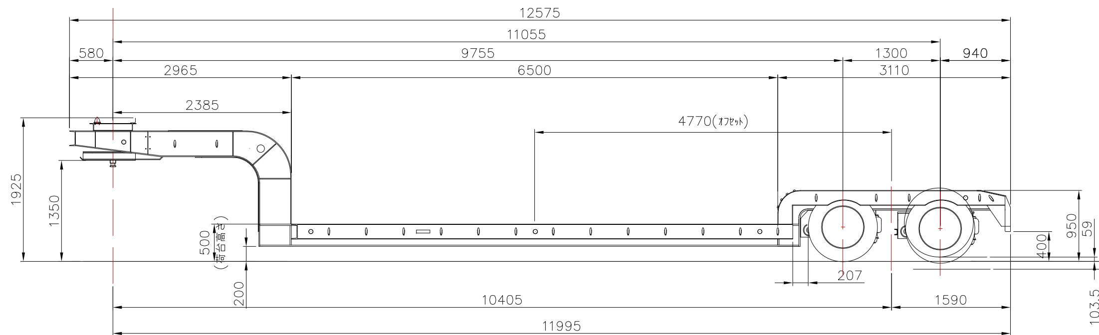
ターンテーブル式ステアリングフルエアサストレーラ
